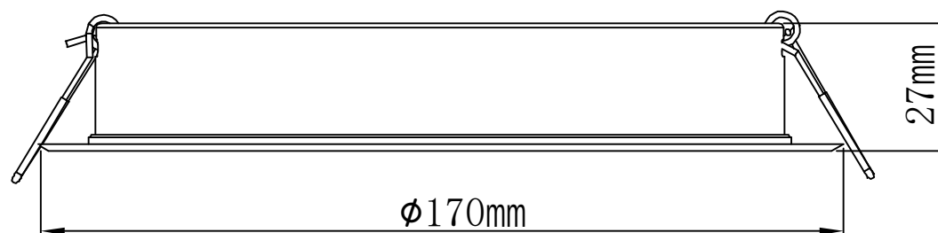
4009-18W-暗装 Cut Out: \phi 150
